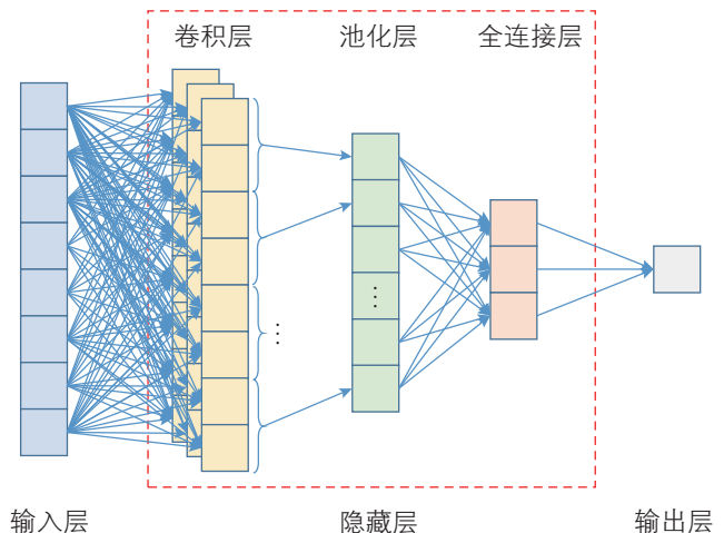
图 3 卷积神经网络结构 Fig. 3 Convolutional neural network structure
